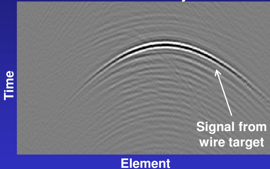
Ultrasound Array Data
